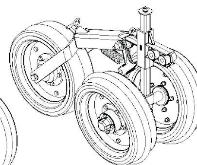
Carrinho cpl da roda compactadora convexa Código: 5124010341-2
