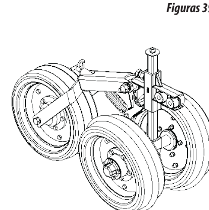
Carrinho cpl da roda compactadora concava Código: 5124010051-0
