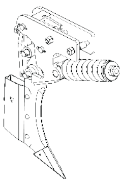
Sulcador c/ desarme e rearme automático Código: 5532010197-1
