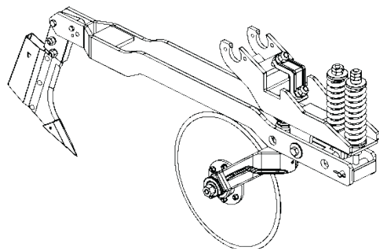
Carrinho maior c/sulcador Código: 5124010531-8
