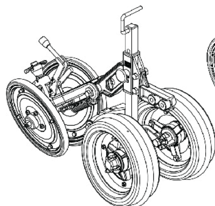
Carrinho da roda de profundidade Excentrica Oscilante e roda "V" Código: 5124010557-1
