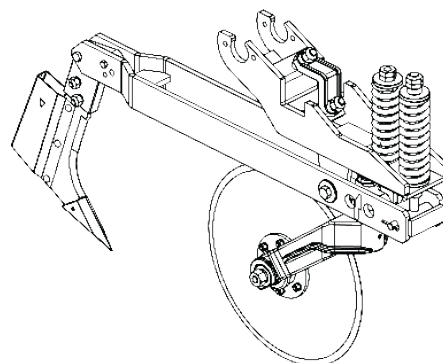
Carrinho menor c/sulcador cpl Código: 5124010530-0
