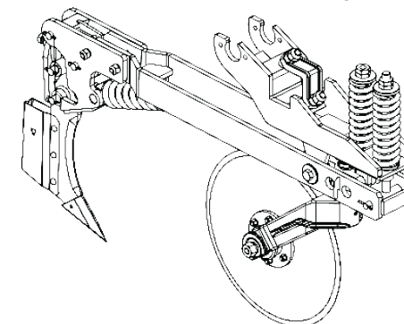
Carrinho menor sulcador automático Código: 5124010609-8
