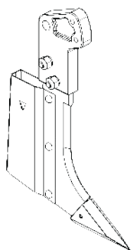
Sulcador c/ suporte Código: 5532010122-0
