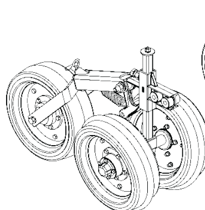
Carrinho cpl da roda compactadora lisa Código: 5124010113-4
