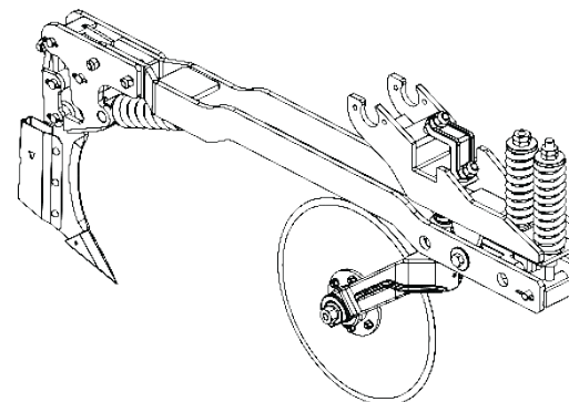
Carrinho maior sulcador automático Código: 5124010610-1
