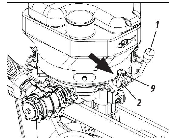
Detalhe "J"
