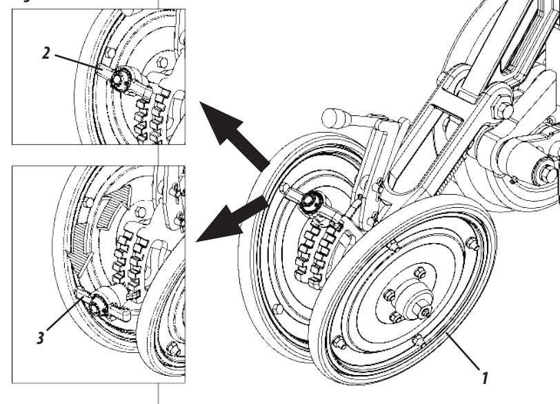
ÂNGULOS DAS RODAS EM "V"
