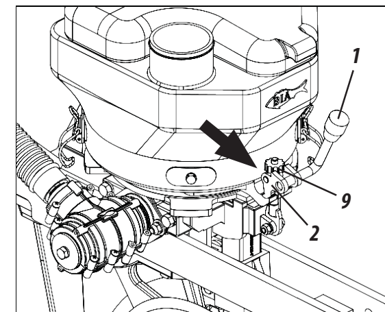
Detalhe "J"
