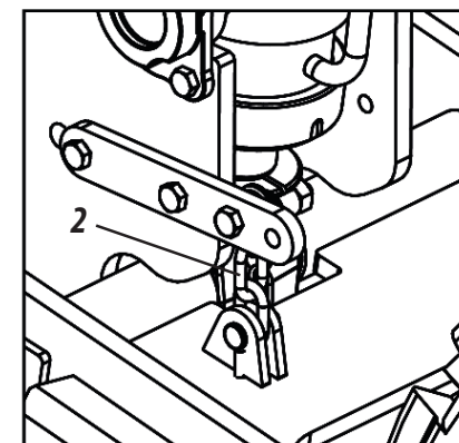
Rodeiro Destravado
