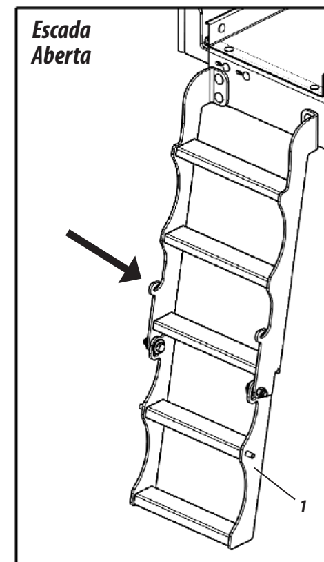
Posição para abastecimento ou manutenção dos depósitos
