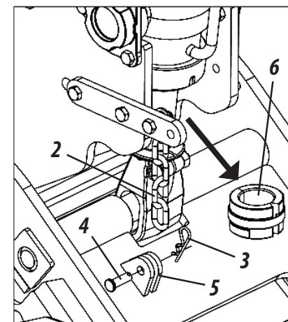
Rodeiro Destravado
