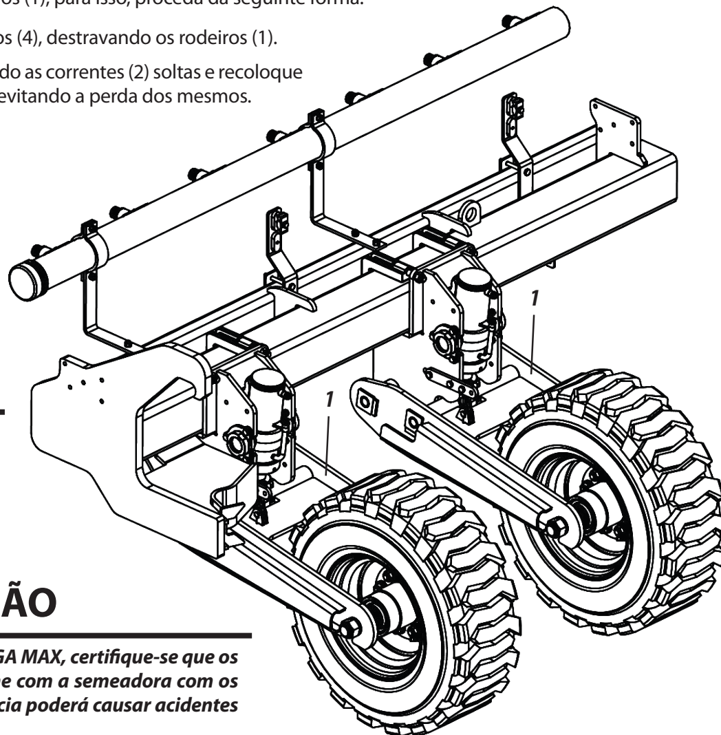
Rodeiro Travado
