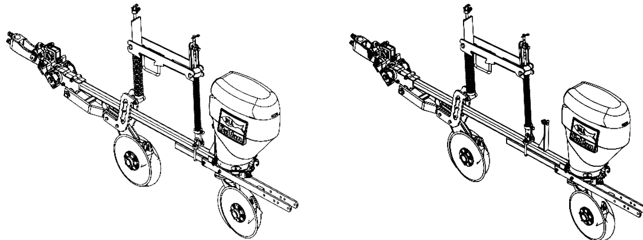
Linha menor direita c/ disco duplo de adubo c/ suporte p/ disco de corte (Sistema Universal 2014)
