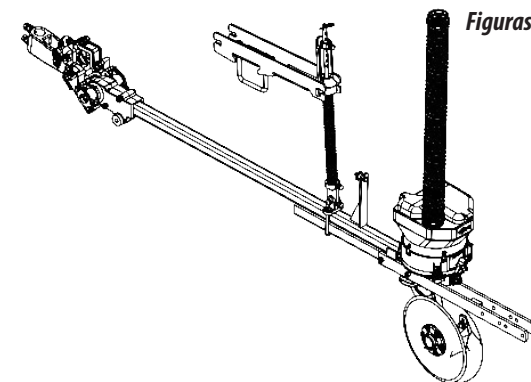
Linha maior esquerda p/ roda oscilante c/ suporte p/ disco de corte p/ 3° depósito (Sistema Universal Titanium 2014) s/ sistema de adubo
