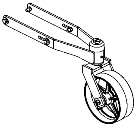
RUEDA DE PROFUNDIDAD COMPLETA CON RODAMIENTO ( MODELO RP/RPU )
