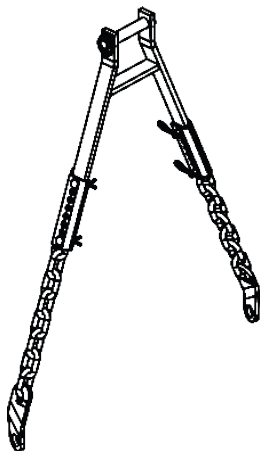
ENGANCHE LIMITADOR DE ALTURA ( MODELO RP )
