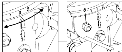
Detalhe "A"
