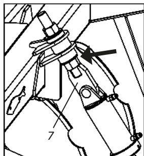
DETALLE "A"
