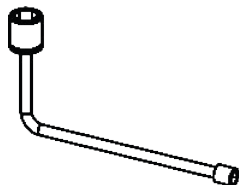
LLAVE "L" P/ TUERCA HEXAGONAL DE 5/8" Y 1.1/4"
