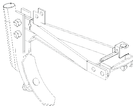
Soporte con pico riscador para fertilización profunda
