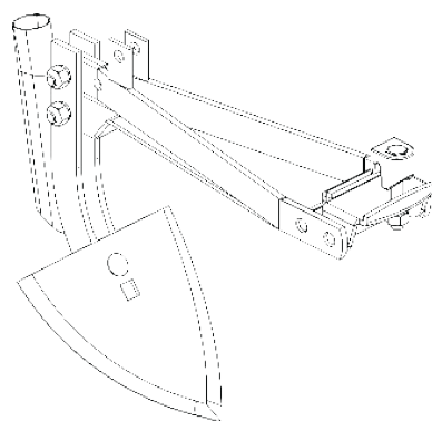
Soporte con pico surcador para plantío de maíz
