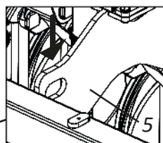
ENGATES DIANTEIROS
