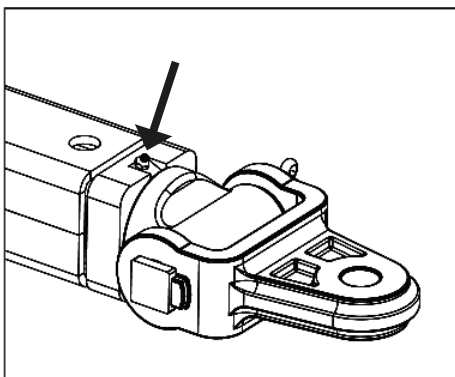
NVCR 48/52/56 DISCOS ESPAÇAMENTO DE 175 MM
