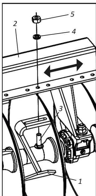
NVCR 28 À 56 DISCOS ESPAÇAMENTO DE 175 MM
