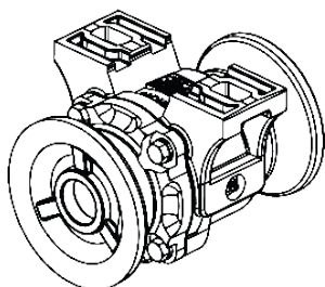
MANCAL A GRAXA - SEM PROTEÇÃO ESPAÇAMENTO 175 MM E 200 MM NVCR 28 A 56 DISCOS
