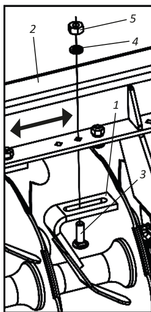
NVCR-E 44 DISCOS ESPAÇAMENTO DE 200 MM
