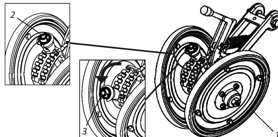
ÂNGULO DAS RODAS EM “V”
