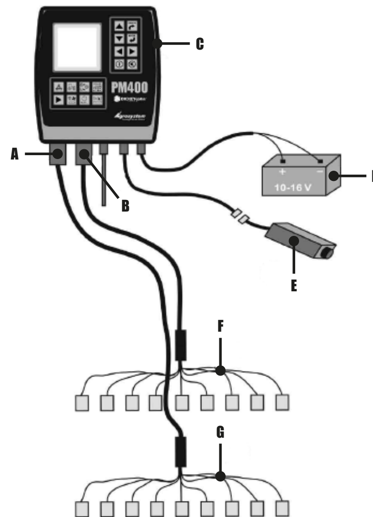
ESQUEMA DE INSTALAÇÃO DO MONITOR
