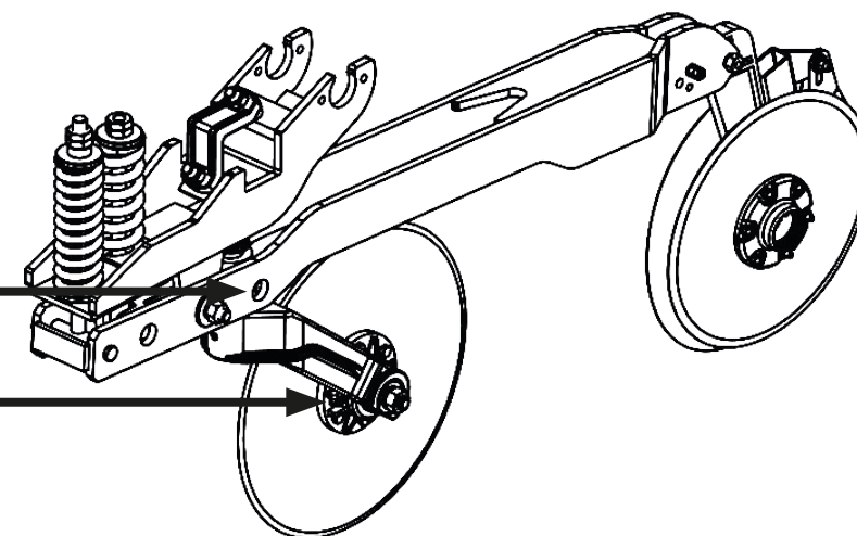
LINHA DO ADUBO MAIOR
