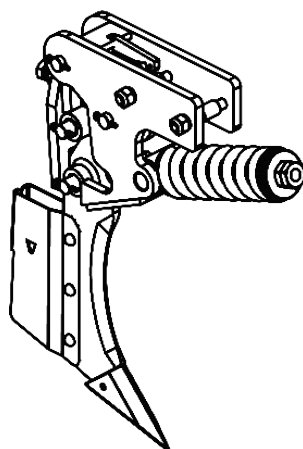
SULCADOR DESARME E REARME AUTOMÁTICO
