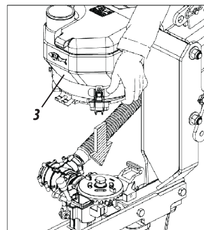
Detalhe "I"
