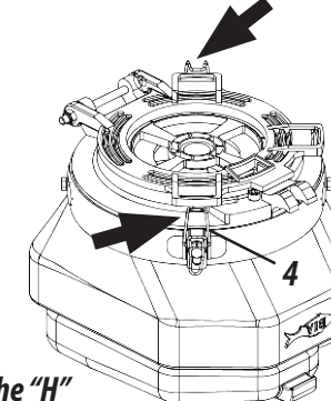
Presilhas
