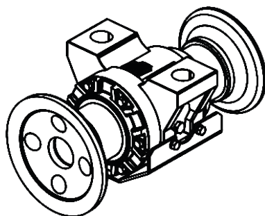
MANCAL AXIAL COM PROTEÇÃO
