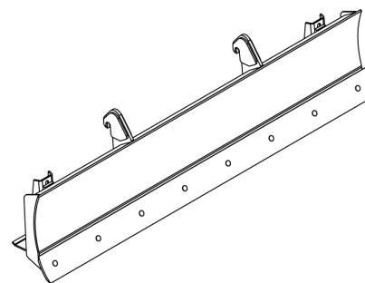
Hoja 2400mm - 5340010028-0 2600mm - 5340010037-0 Ver página 58
