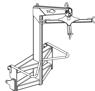
Cabrestante 2547260205-8 Ver página 58
