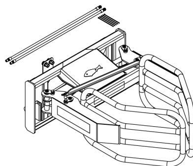
Bifurcación Bale 5304010013-6 Ver página 55
